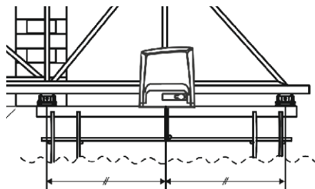
Рис. 4. Место установки привода
