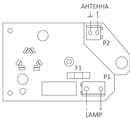
Рис. 21. Схема подключения сигнальной лампы RT-LA230V
