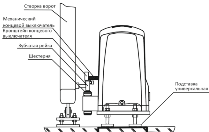
Рис. 10. Схема установки привода с механическими концевыми выключателями
