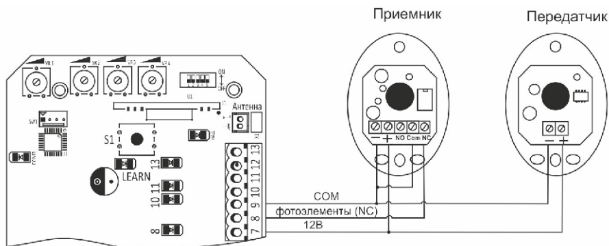
Рис. 20. Схема подключения фотозадающих элементов RT-F1
